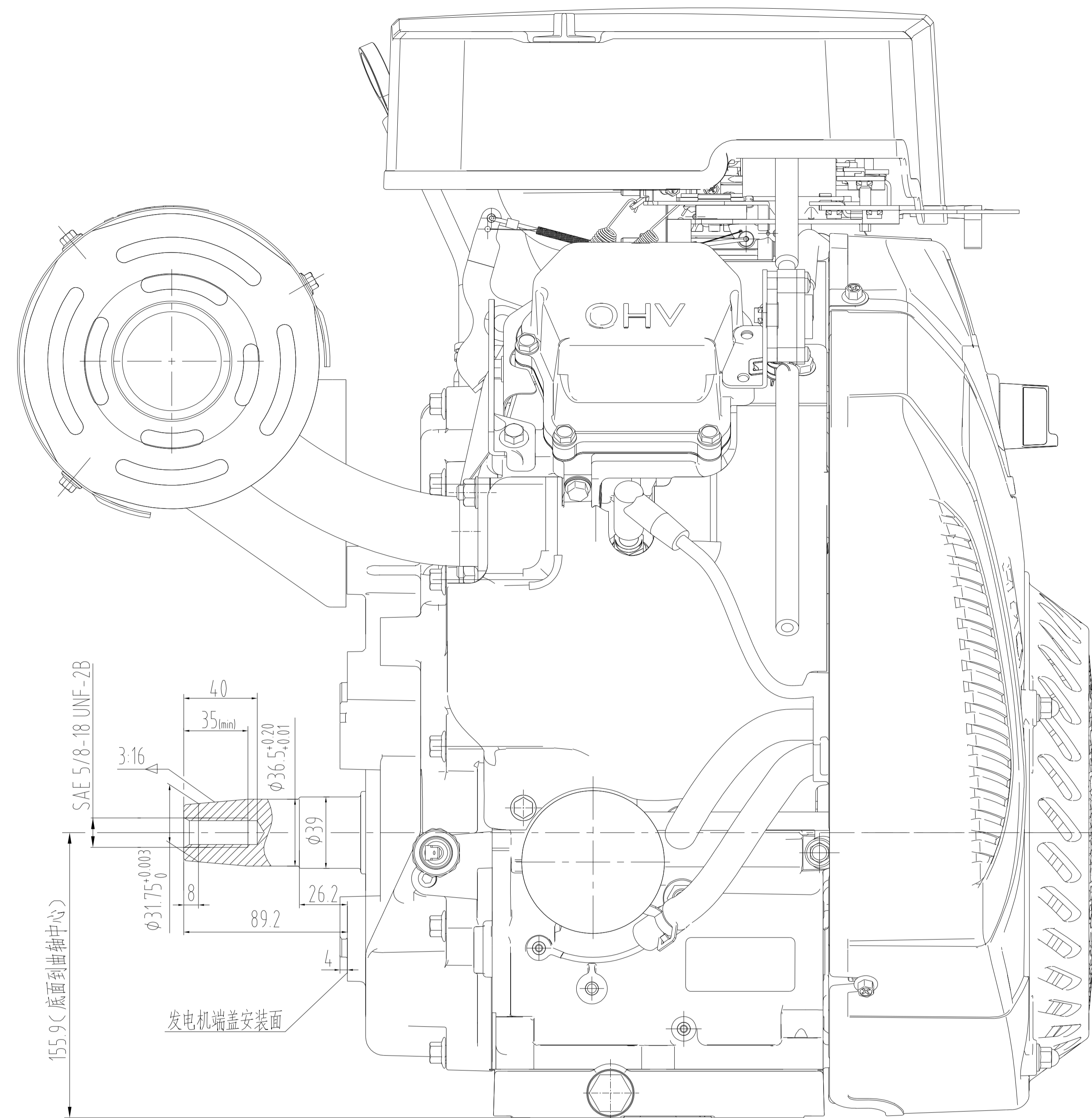
发电机状态
