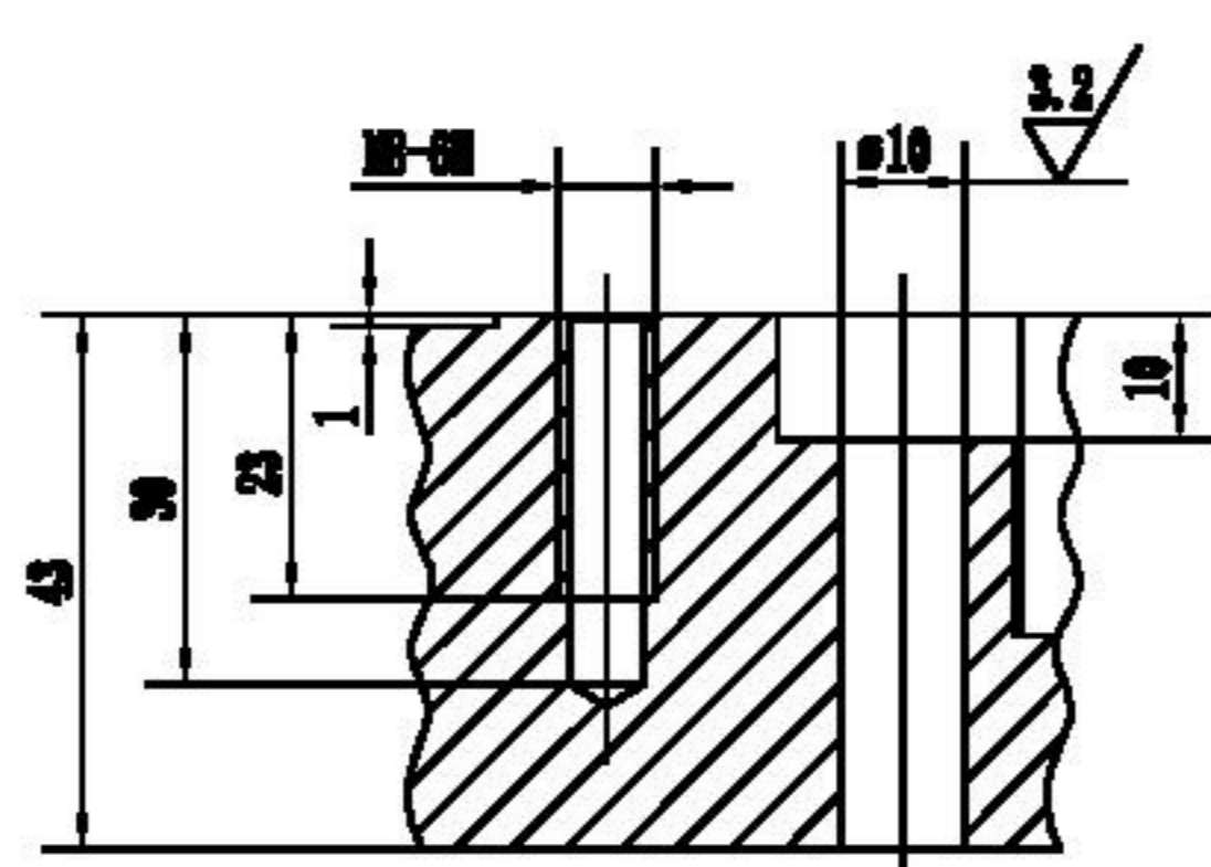
R-R 旋转
