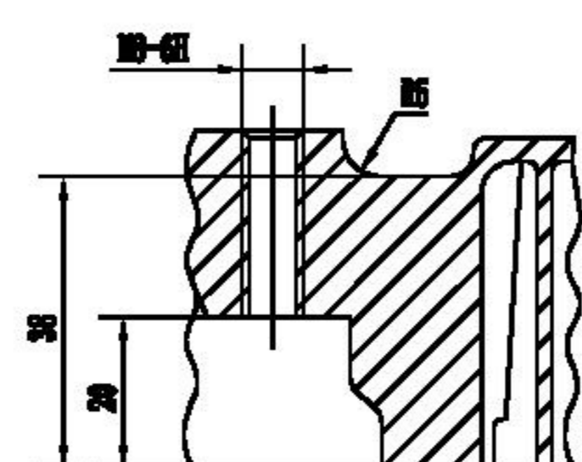
O-O 略画
