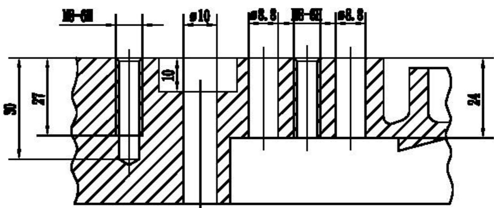
G-G 旋转
